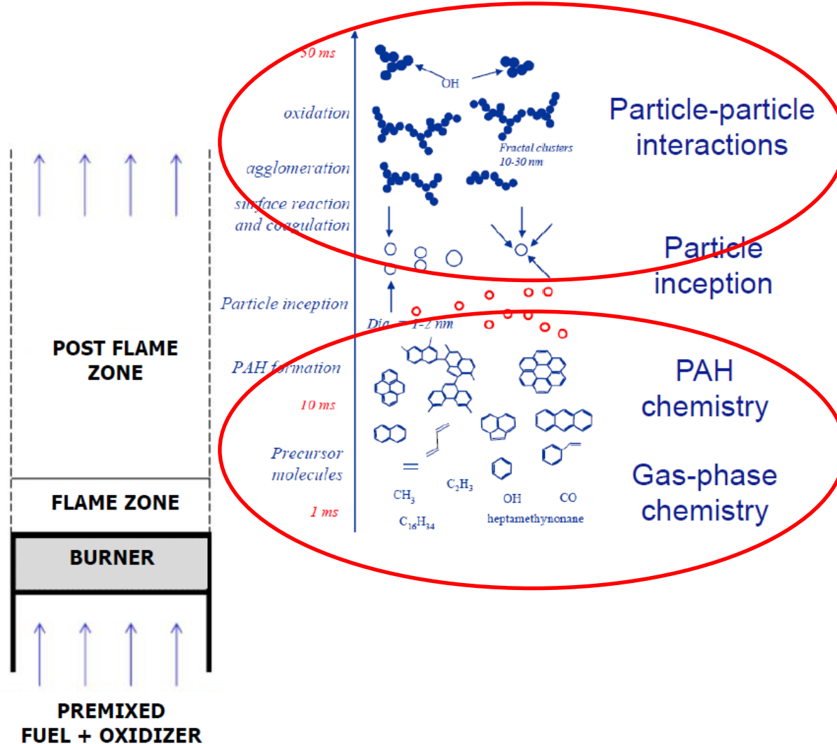
benzene
